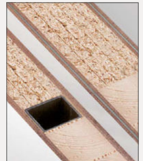
Klimaklasse III mit Stahlrohrverstärkung oder Aluminiumverbundabspernung
