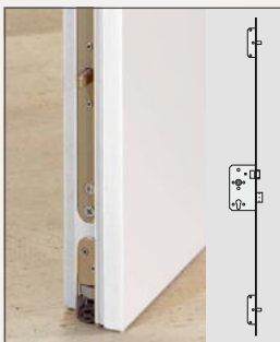
Dreifachverriegelung, Bodendichtung und Türaufschlagdichtung
